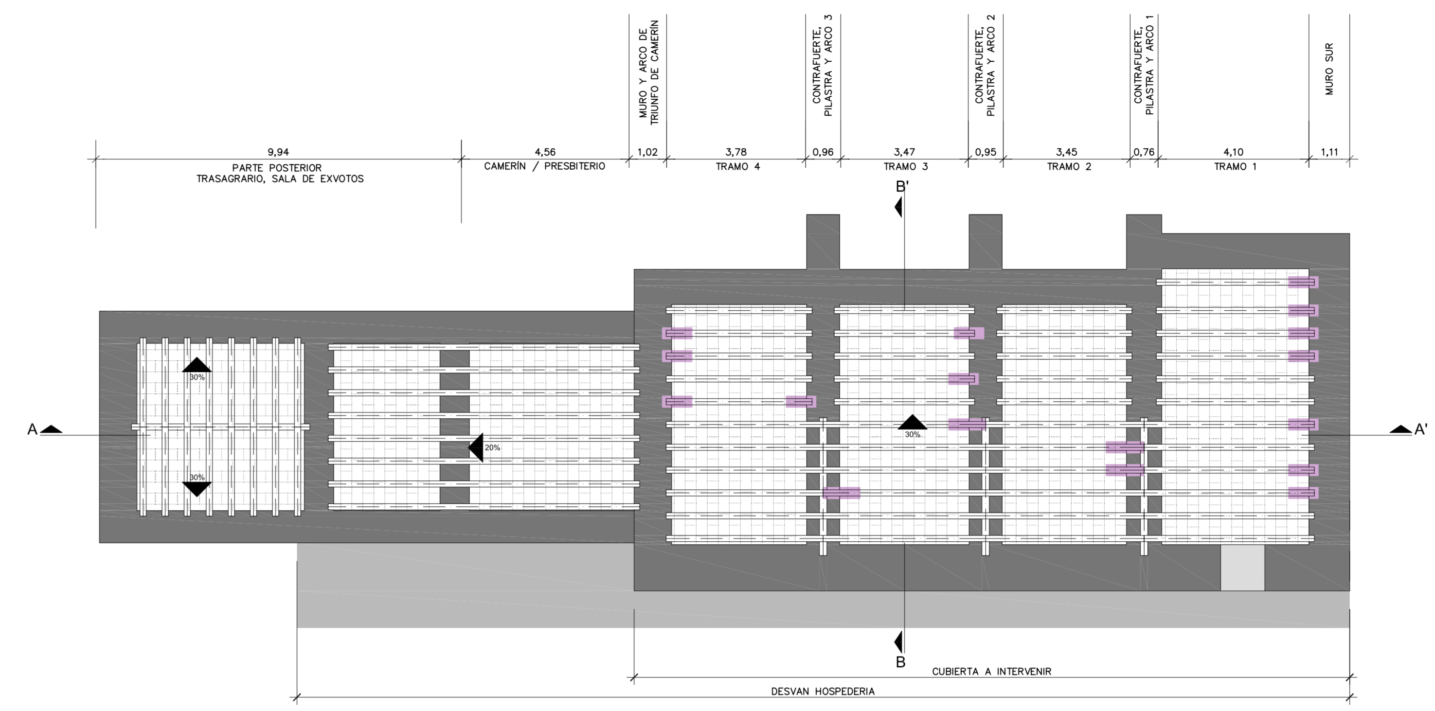
ESTRUCTURA COBERTA
