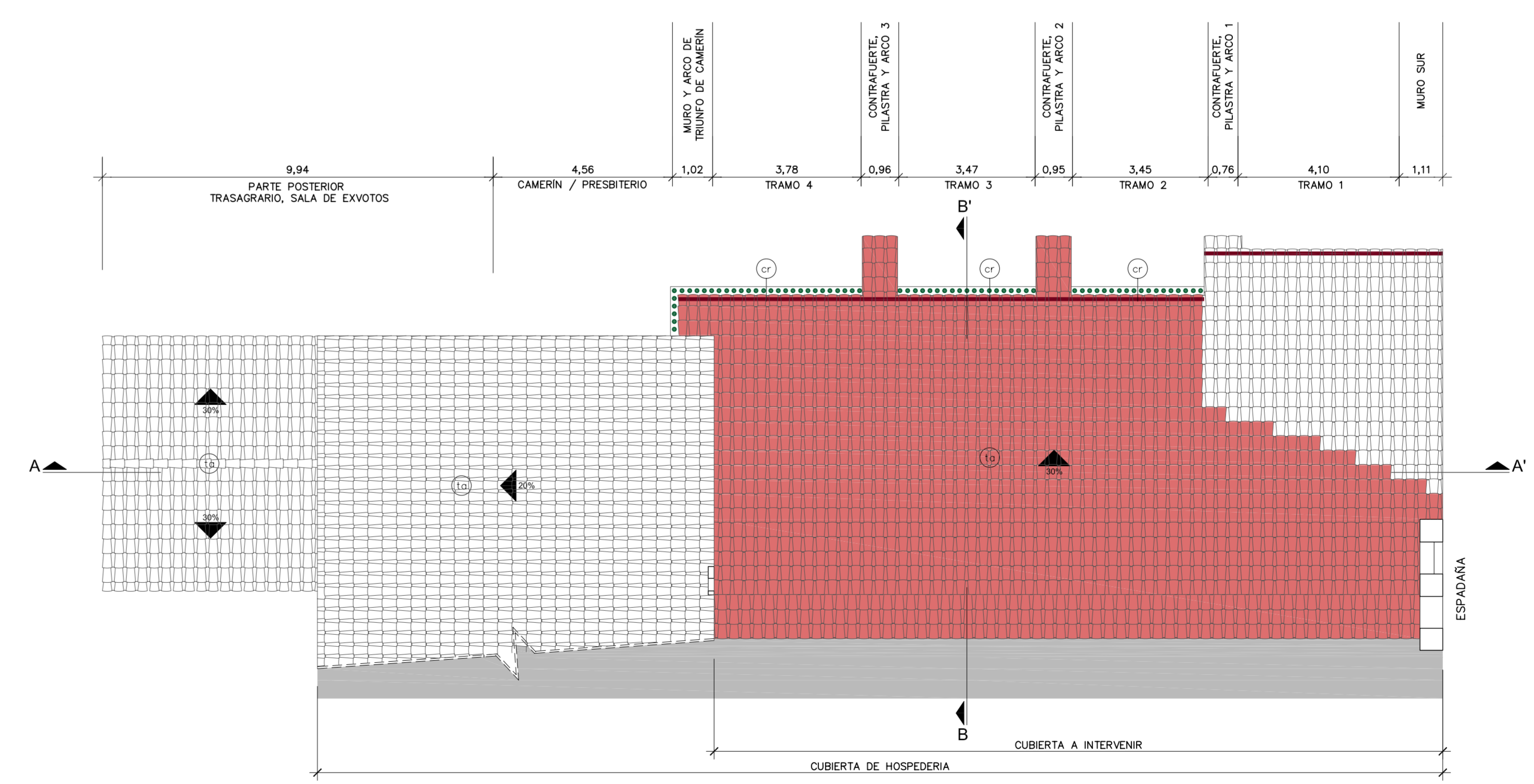
PLANTA COBERTA
