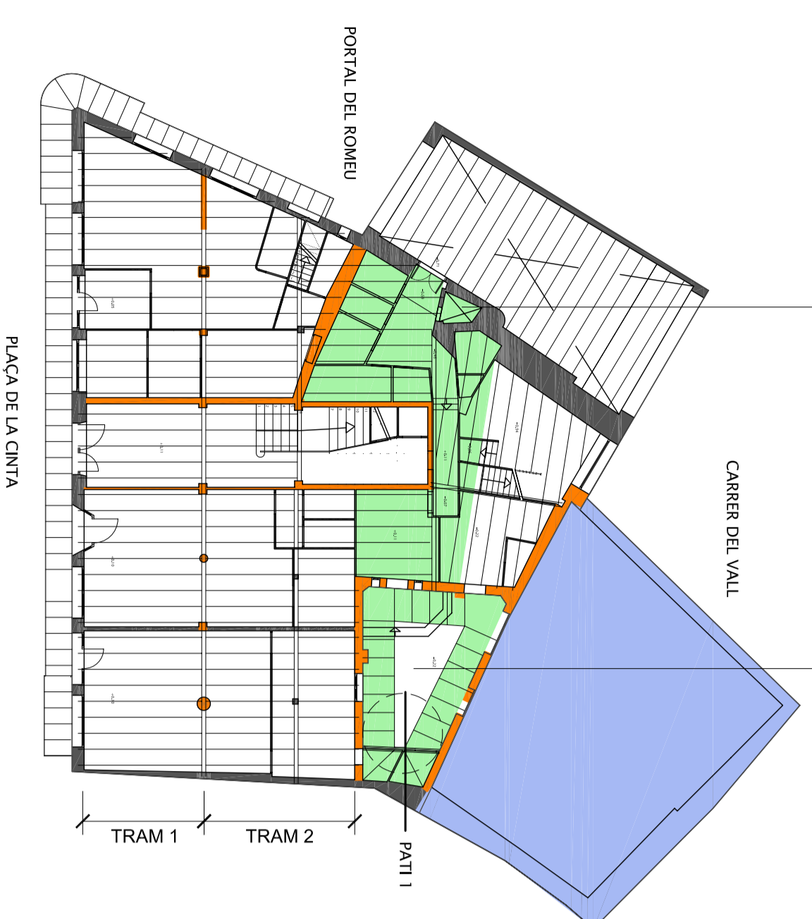
SOSTRE 1 (+5,06)
