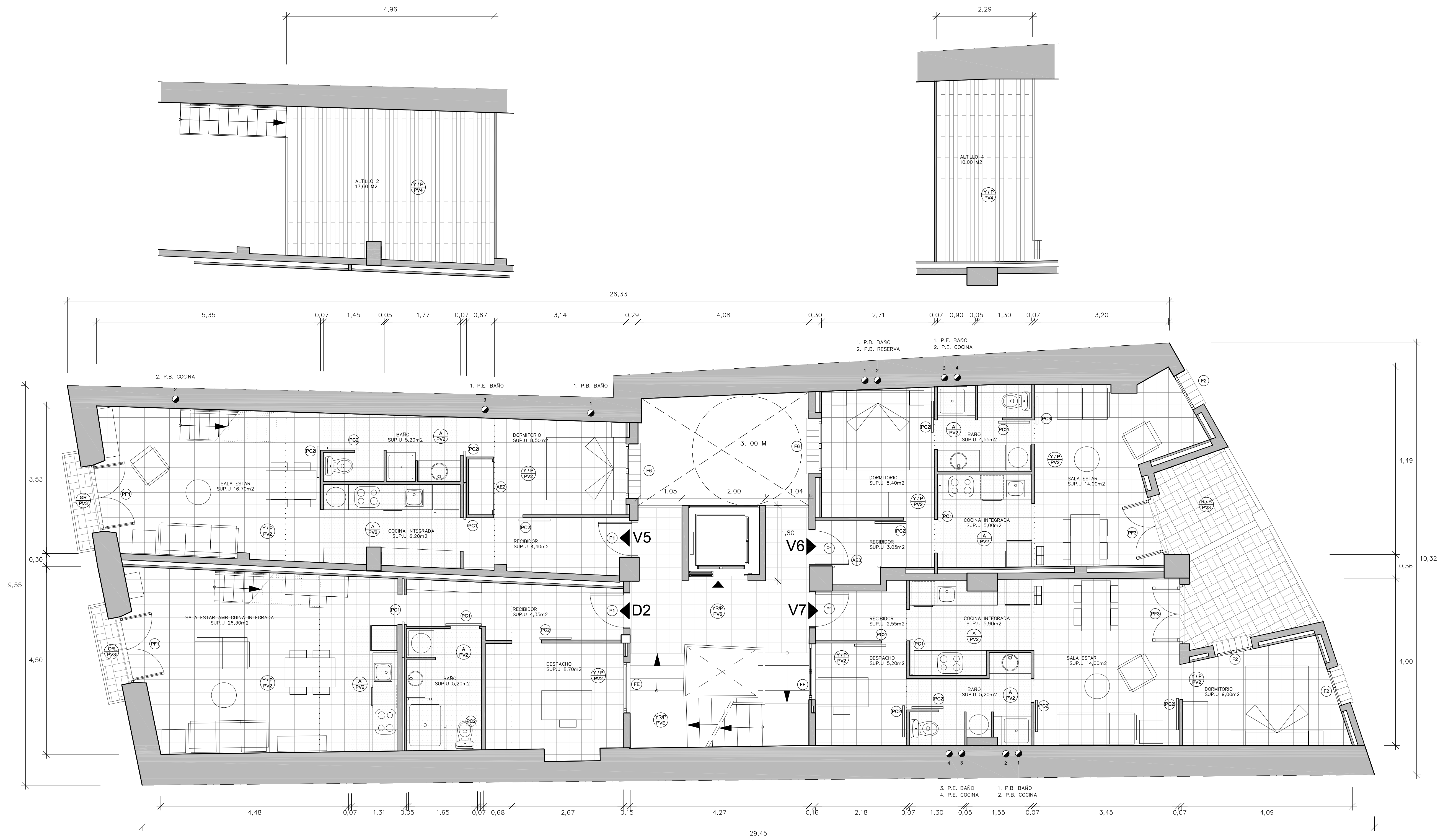
PLANTA PRIMERA
