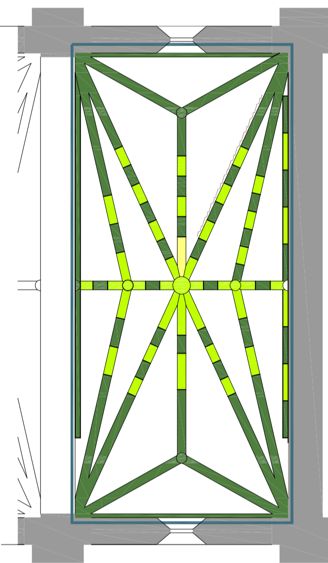
PLANTA TRAMO 3
