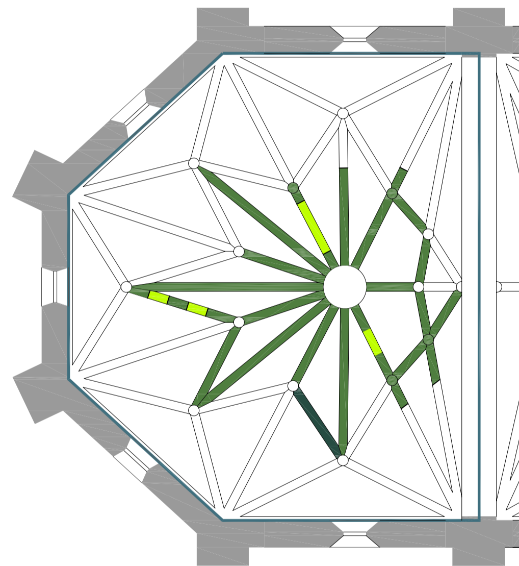
PLANTA PRESBITERIO
