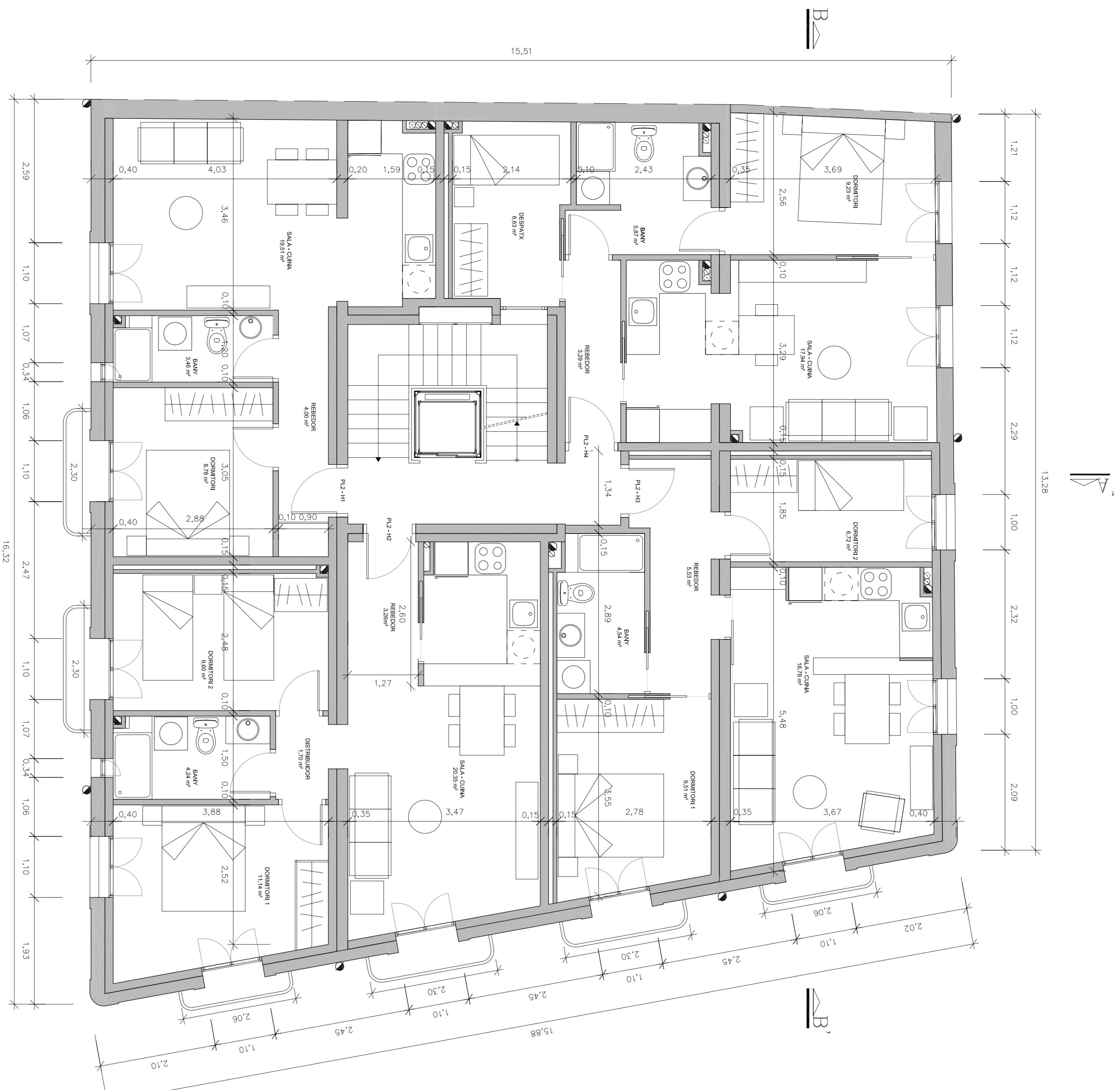
PLANTA SEGONA
