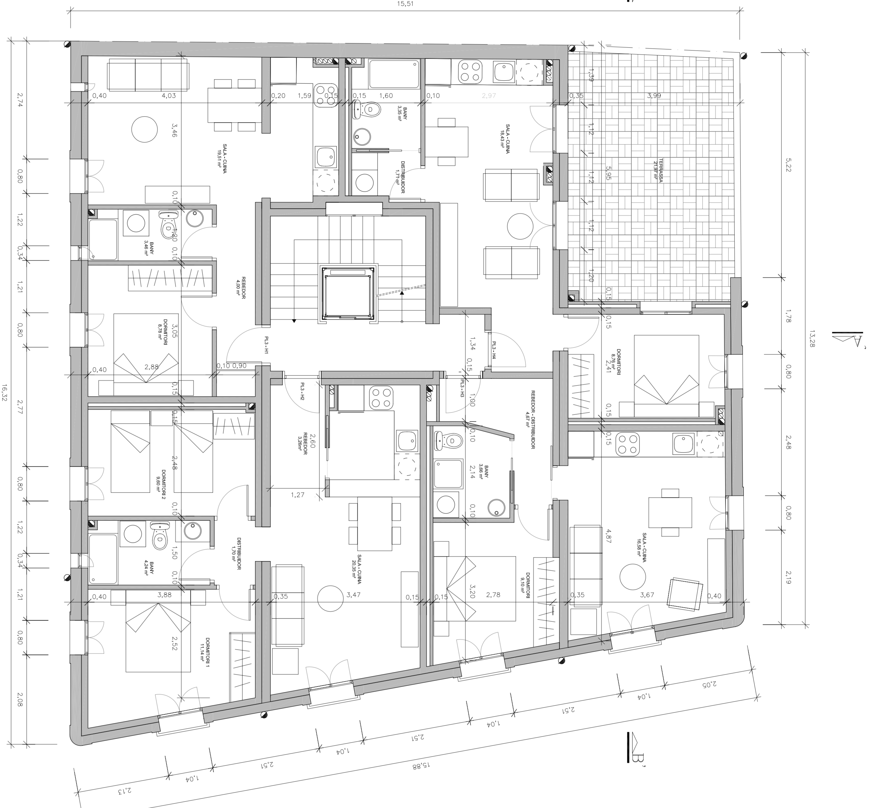
PLANTA TERCERA
